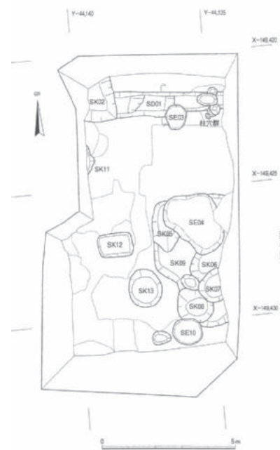
図9 ST13-5次調査地平面図
