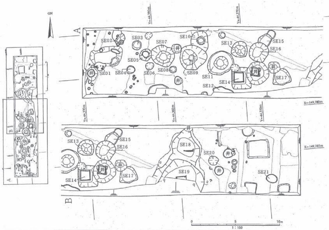
図22 CU98-1次調査地平面図
