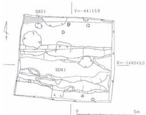
図11 ST96-7次調査地平面図
