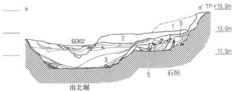
図7 ST96-4次調査地断面図
