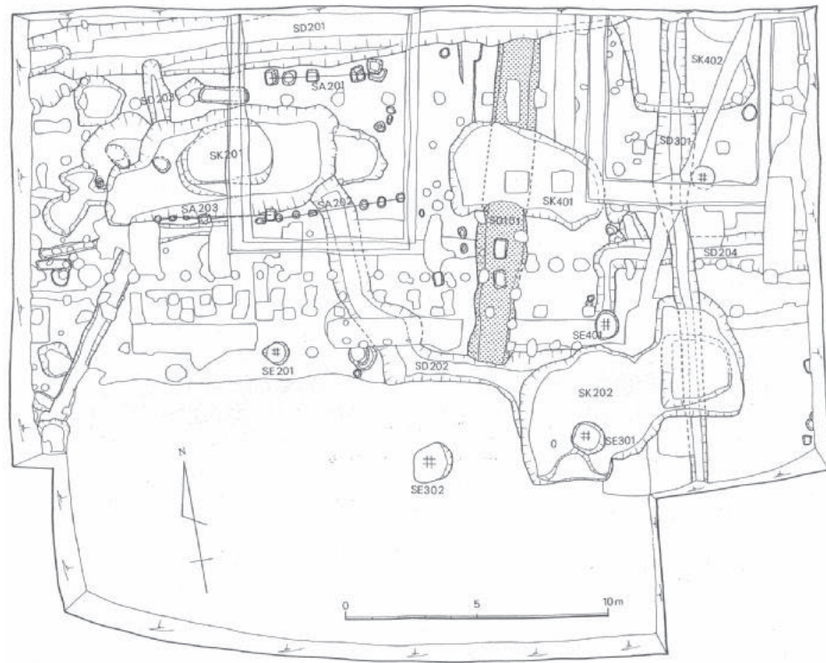
図12 ST85-1次調査地平面図
