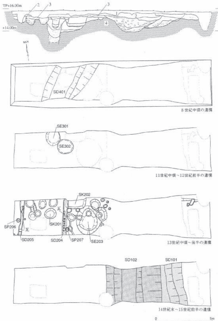
図5 ST99-5次調査地平面図
