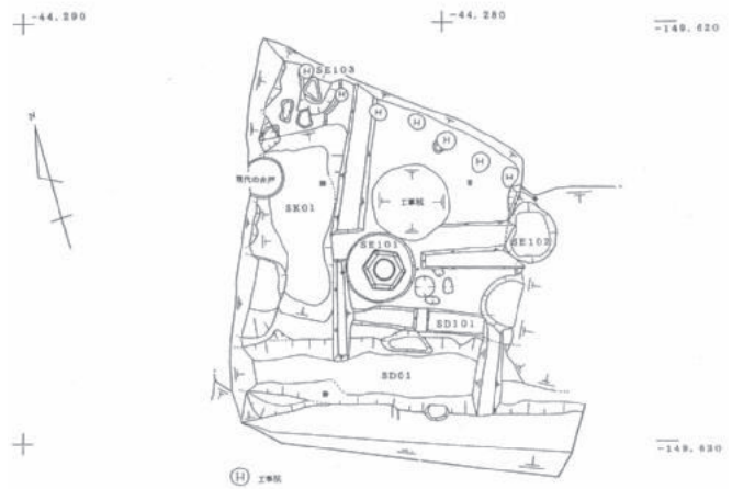
図20 ST92-7次調査地平面図
