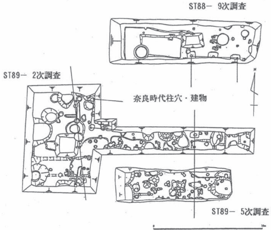
図15 ST88-9・89-2・89-5次調査地平面図
