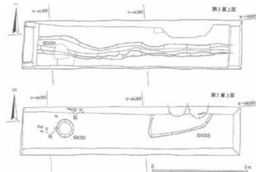
図10 ST15-1次調査地平面図
